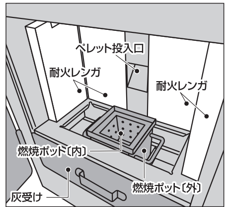
内部図
