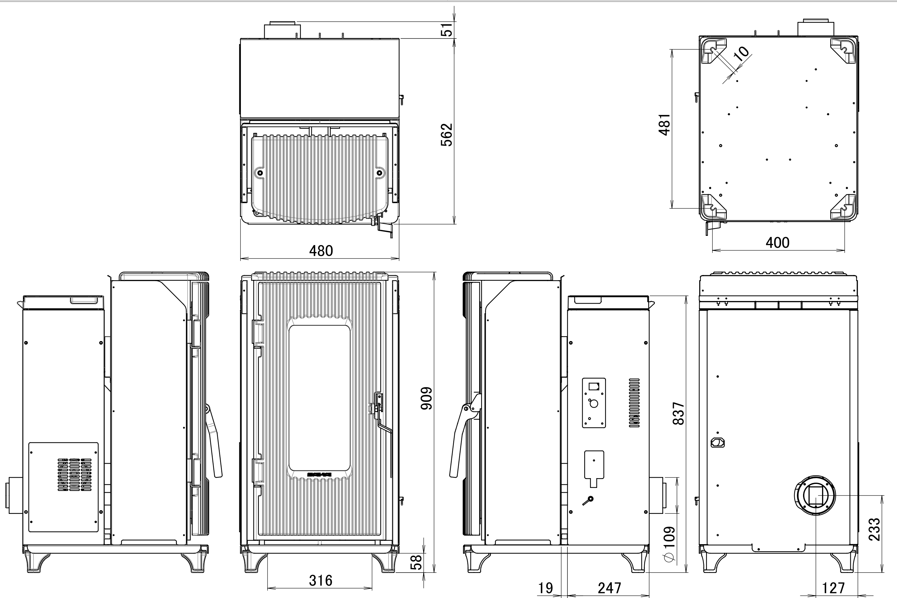
SAIKAI RS-4 外觀寸法図
